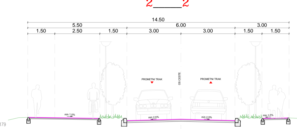
NORMALNI POPREČNI PROFIL 2-2
